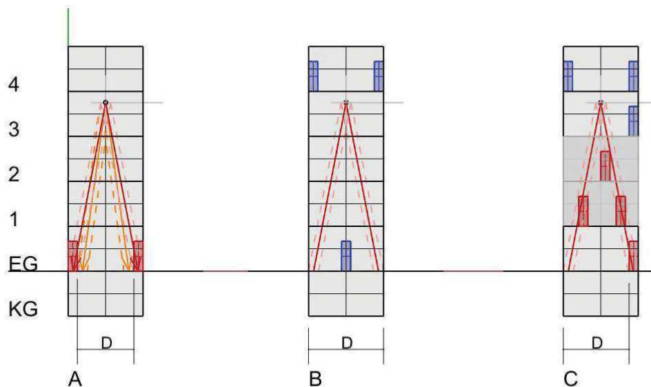
Abbildung 1.3 – Öffnungen in Mauerwerksscheiben
