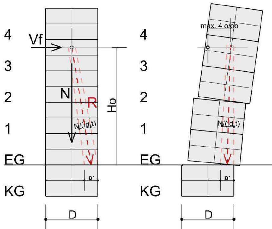
Abbildung 1.1 – Umkippen und Gleiten einer Mauerwerksscheibe
