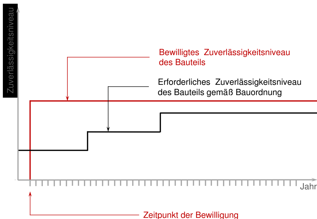
Abbildung 2: Darstellung verschiedener Zuverlässigkeitsniveaus von Bauteilen
