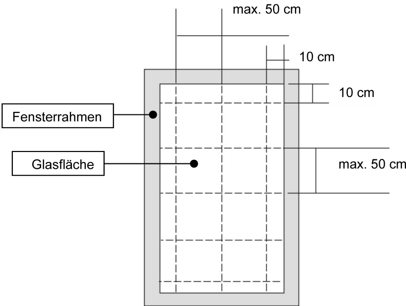
Bild 4 — Messraster (Skizze)
