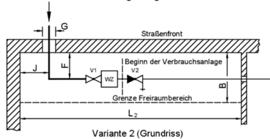
Variante 2 - Wasserzähleranlage abgewinkelt zur Anschlussleitung
