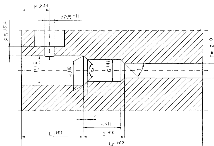
Bild 1: Abmessungen des Meßlaufes
