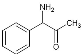
1-Amino-1-Phenylpropan-2-on
