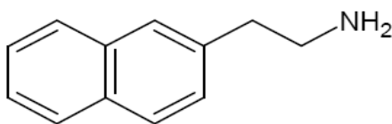
2-(Naphthalen-2-yl)-Ethanamin
