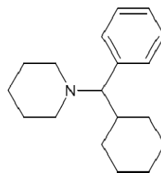
1-[Cyclohexyl(Phenyl)methyl]-Piperidin
