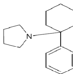
1-(1-Phenylcyclohexyl)-Pyrrolidin
