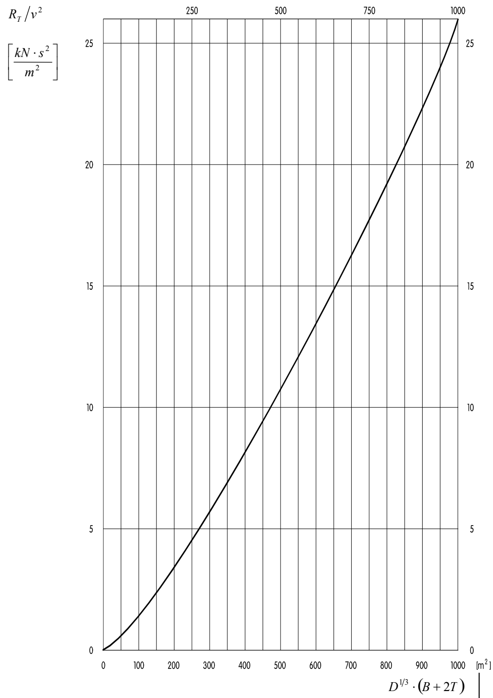
Tafel 3: Diagramm zur Ermittlung von R_T/v^2 in Abhängigkeit von D^{1/3} \cdot (B + 2T)
