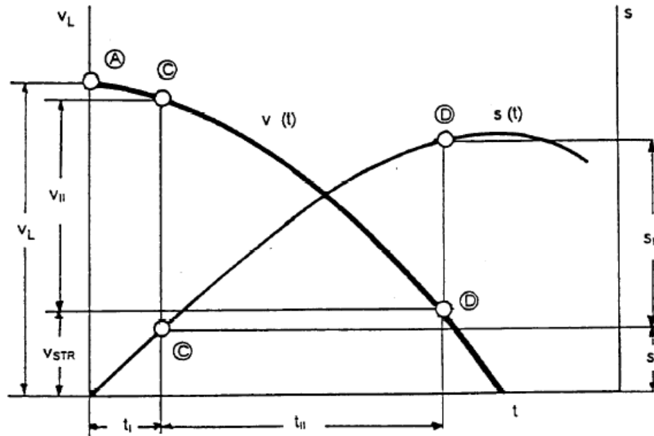
Bild 1 Stoppwege
