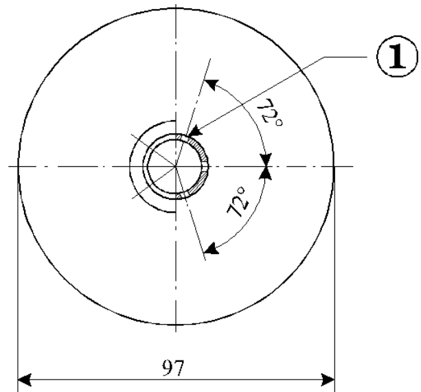
Abb. 3: Hohlter Bronzezylinder, einseitig verschlossen Aufriss und Grundriss
