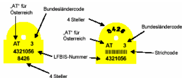
Abbildung 1: Gestaltung der Ohrmarke für Schweine gemäß §§ 7 und 23
