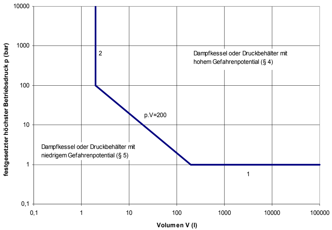
Abbildung 1: überhitzungsgefährdete Dampfessel oder Druckbehälter gemäß § 4 Abs. 3
