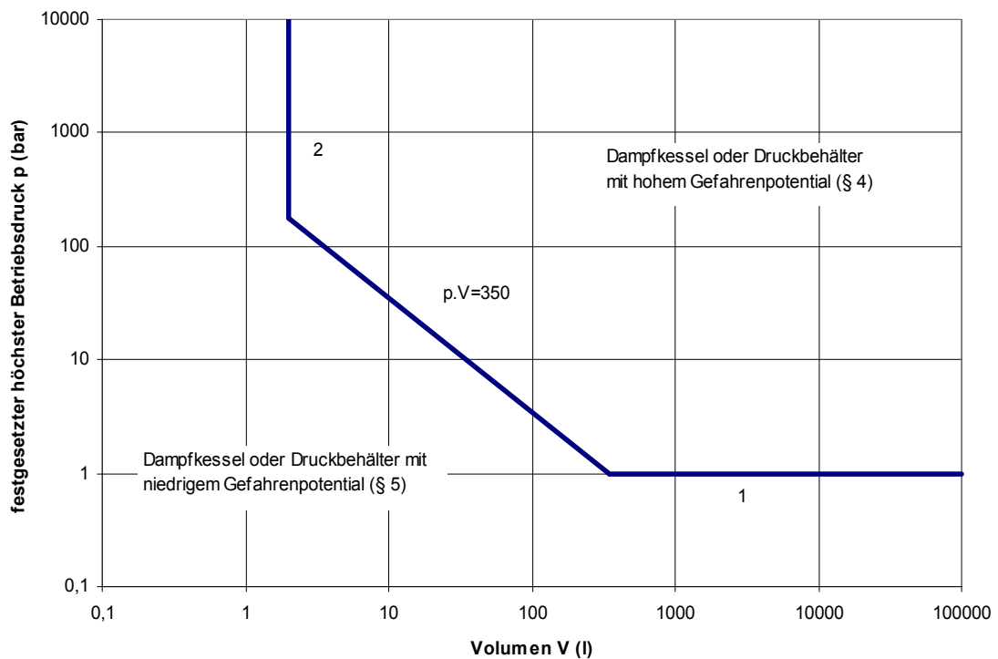
Abbildung 2: überhitzungsgefährdete Dampfessel und Druckbehälter aus Rohren bis einschließlich DN 32 gemäß § 4 Abs. 4
