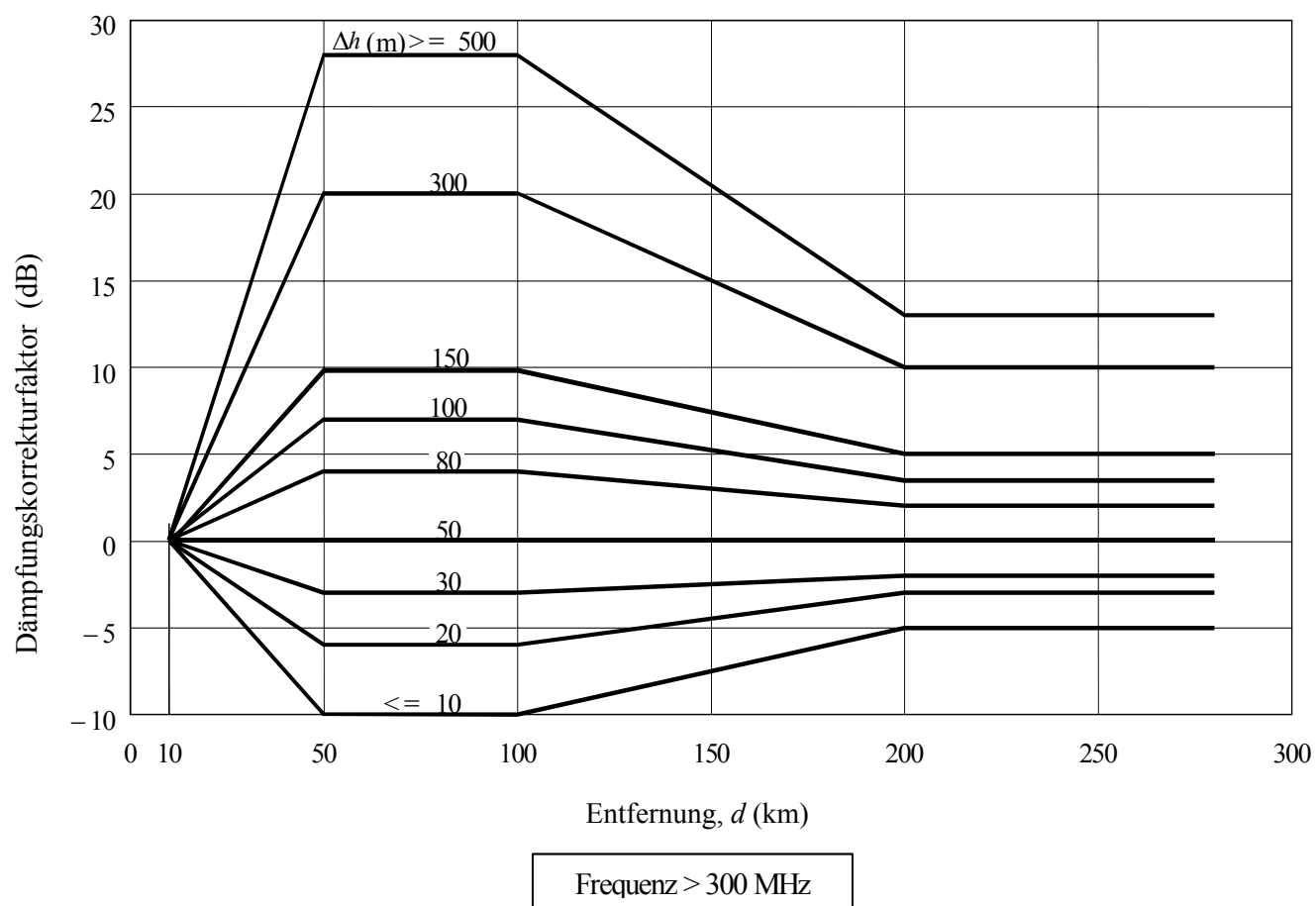
Abbildung 2 - Dämpfungskorrekturfaktor als Funktion der Entfernung d (km) und der Geländerauhigkeit \Delta h (m) für Frequenzen > 300 MHz
